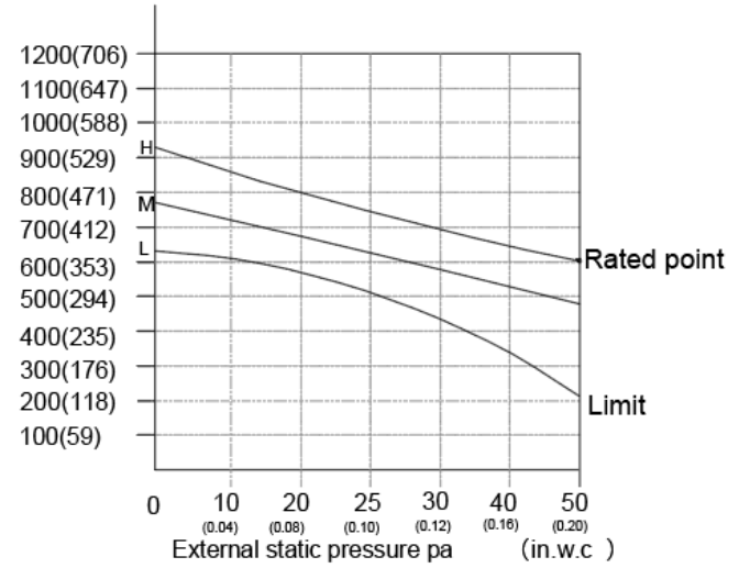
Fig. 14 — Fan Performance - DLFSDAH12XAK
