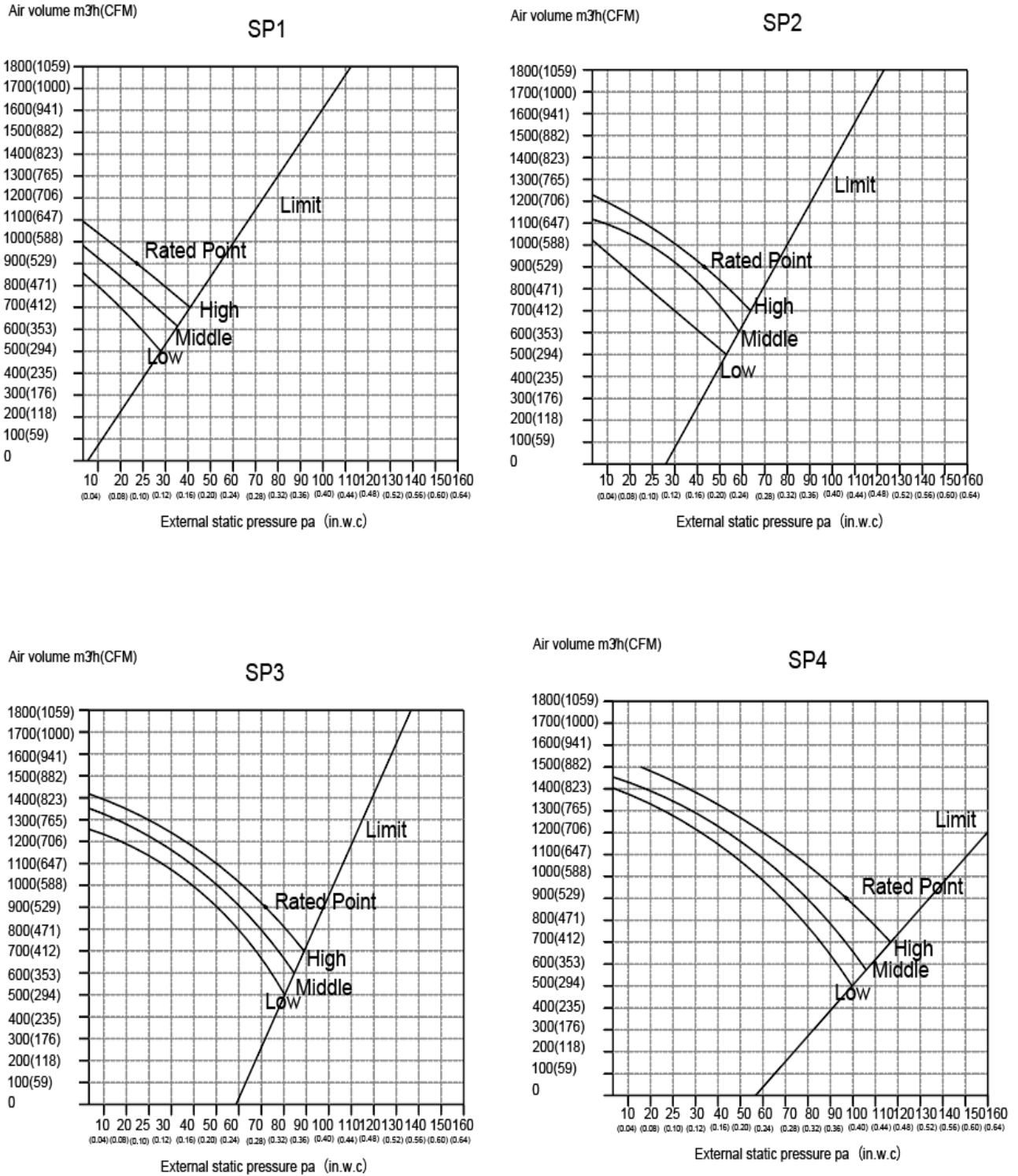
Fig. 15 — Fan Performance - DLFSDAH18XAK
